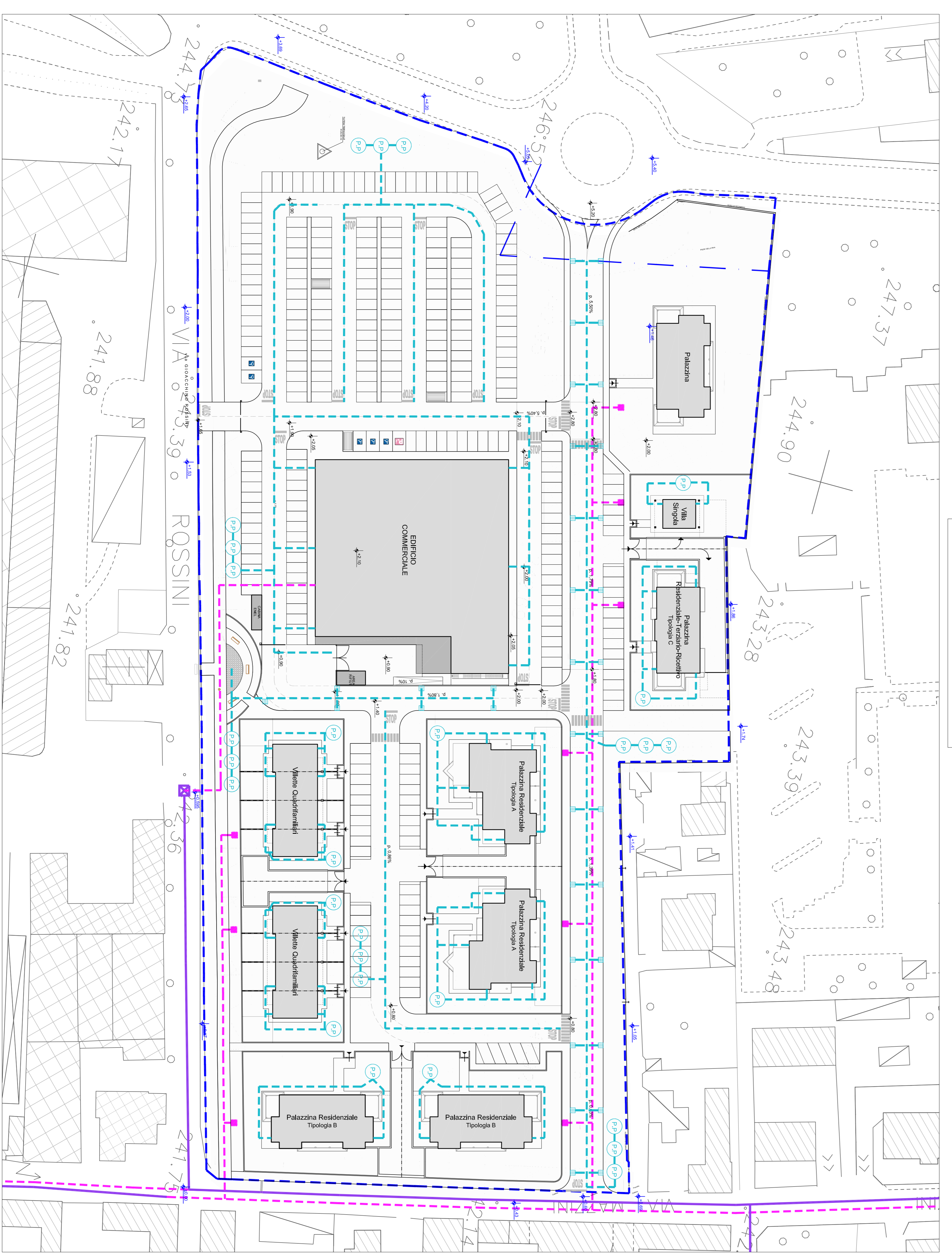
Schema rete fognaria Scala 1:500
