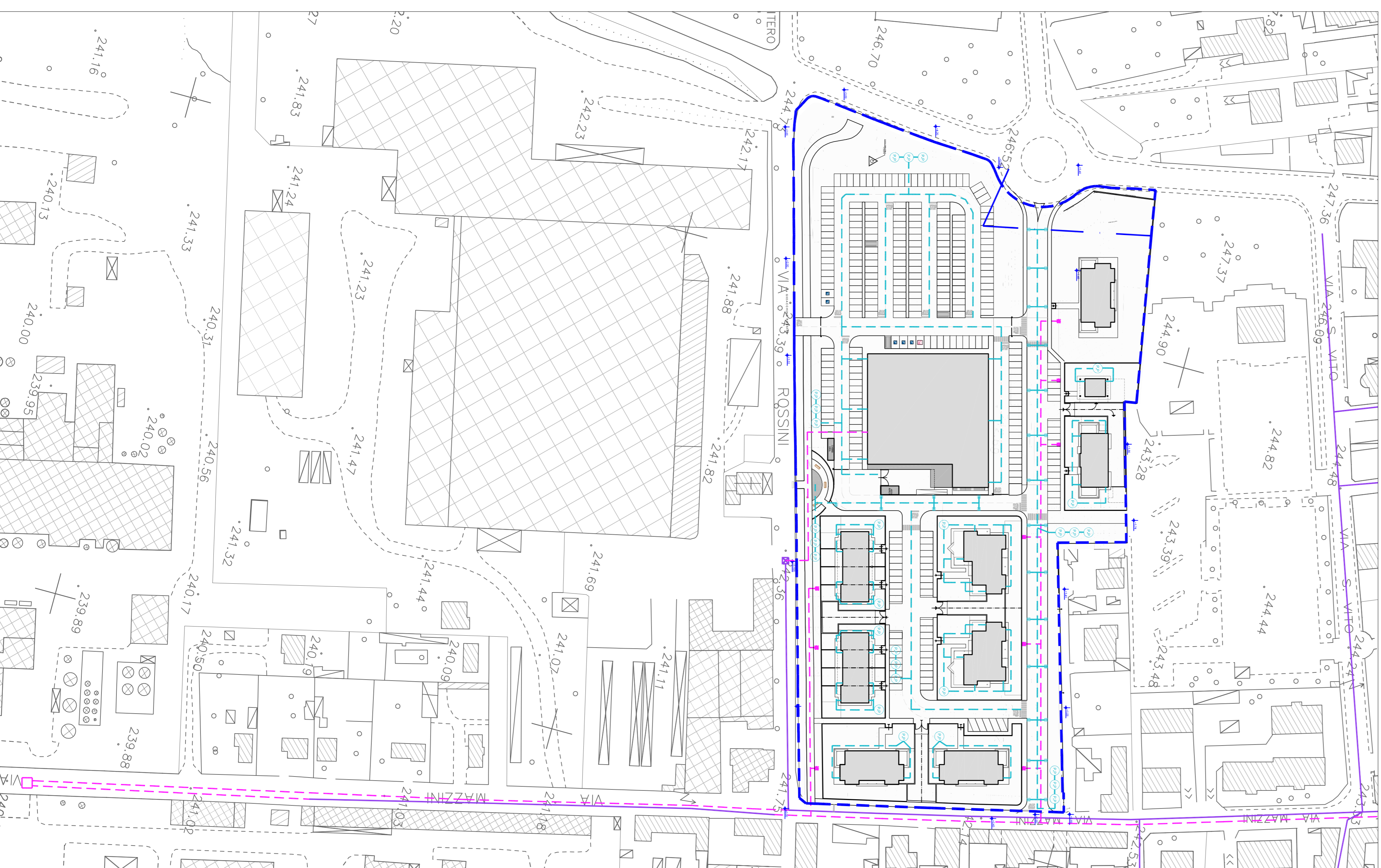
Schema rete fognaria comprensiva del tratto extracomparto su via per Olgiate Scala 1:1'000
