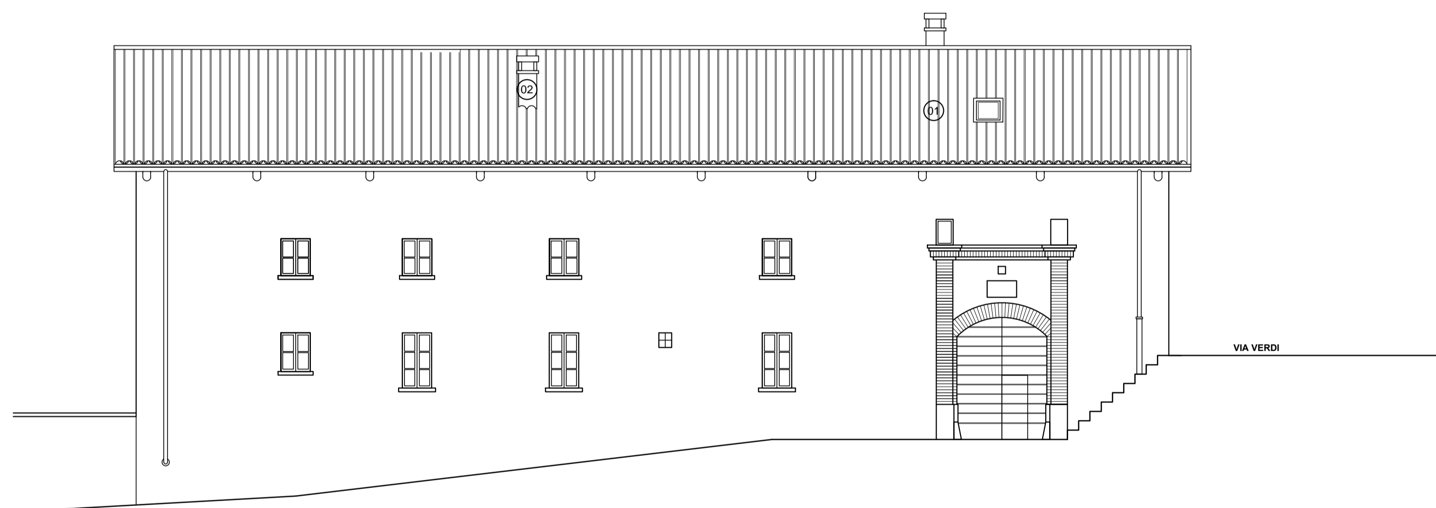
FRONTE NORD
