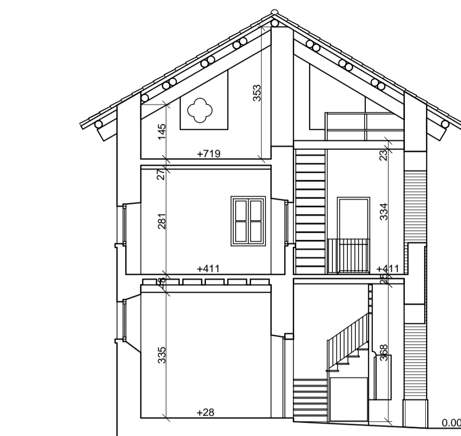
SEZIONE AA
