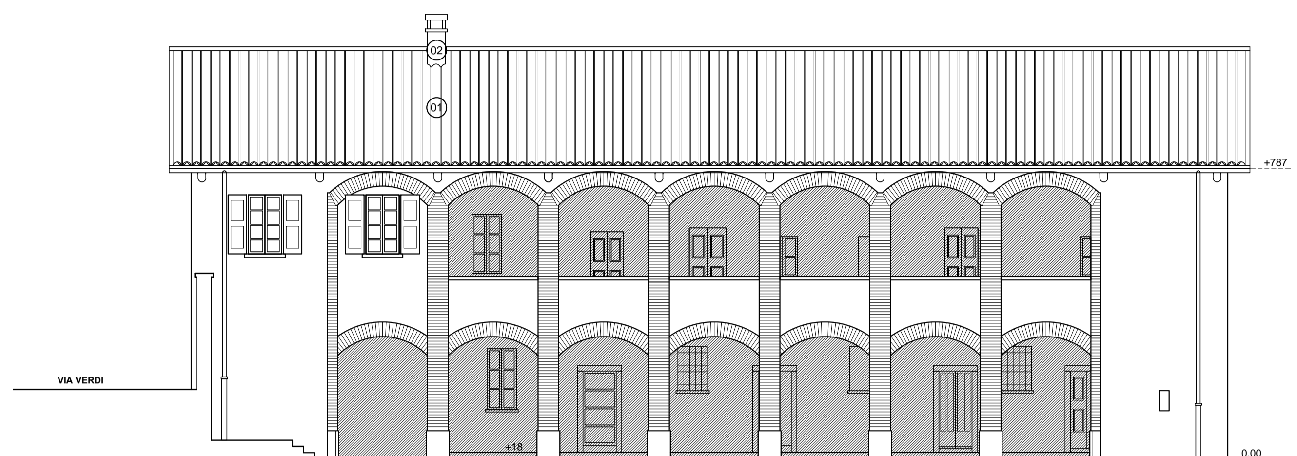
FRONTE CORTILE
