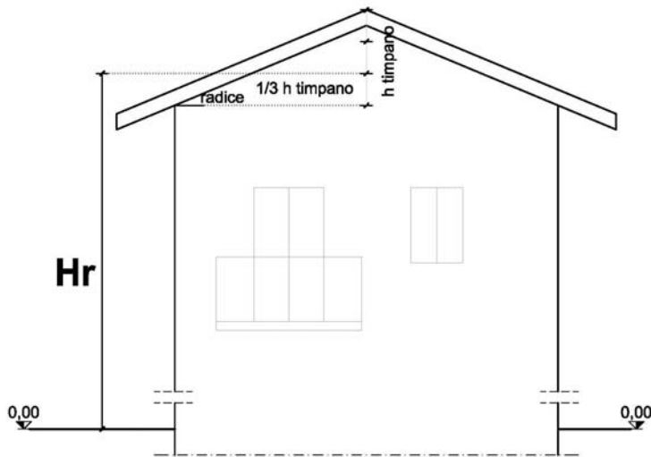
art. 5.12 - Hr, altezza reale edifici residenziali, prospetto a timpano
