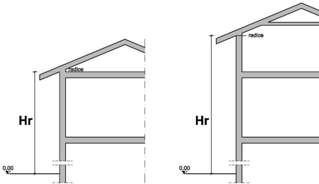
art. 5.12 - Hr, altezza reale edifici residenziali
