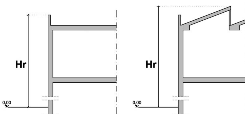
art. 5.12 - Hr, altezza reale edifici produttivi
