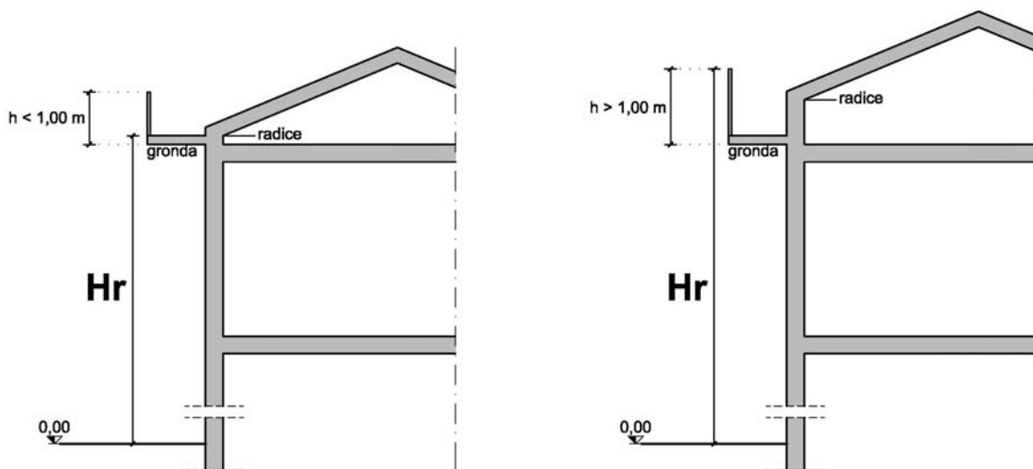
art. 5.12 - Hr, altezza reale edifici residenziali
