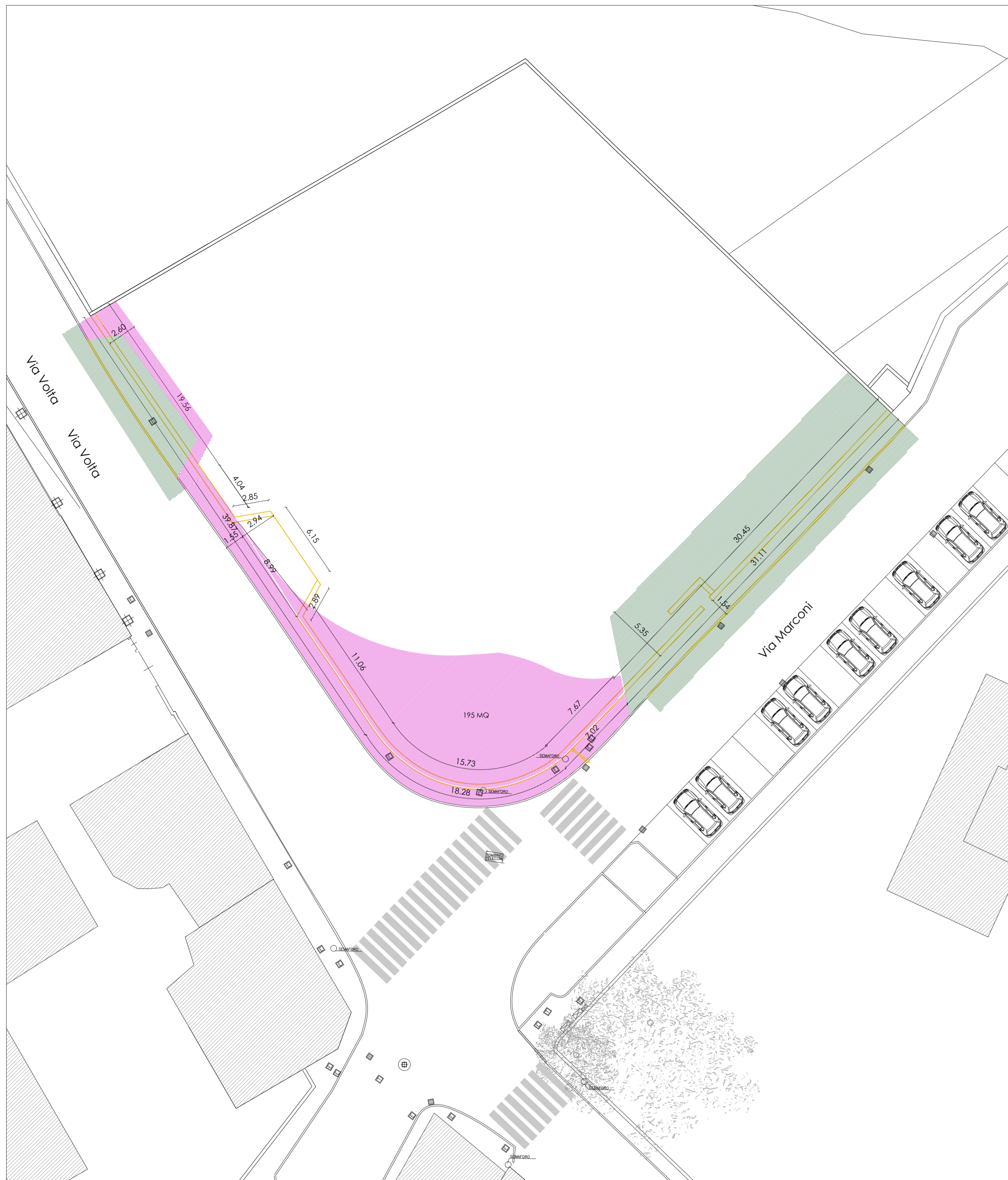
PLANIMETRIA DEMOLIZIONI Scala 1:200
