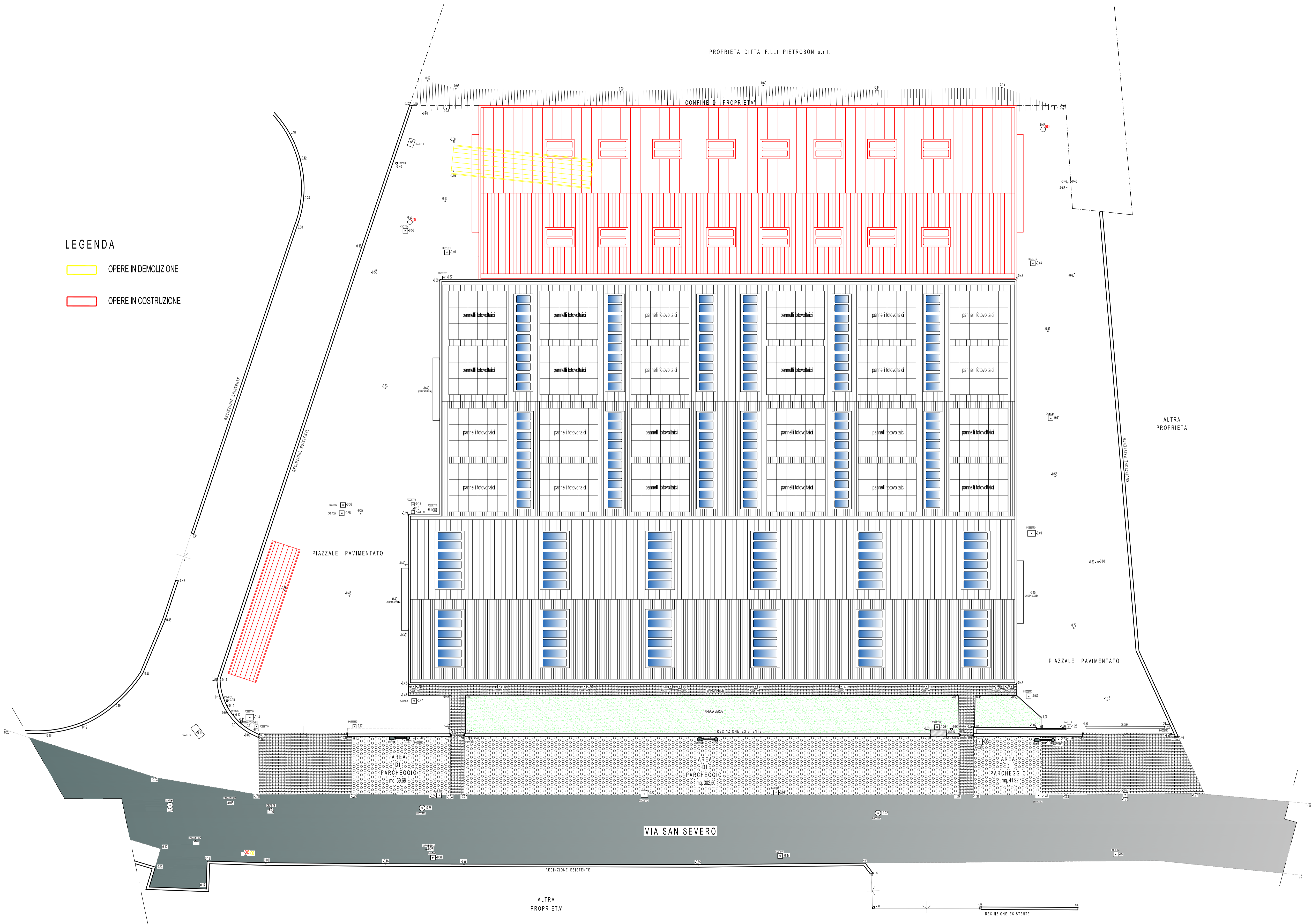
PLANIMETRIA GENERALE DI COMPARAZIONE scala 1:200
