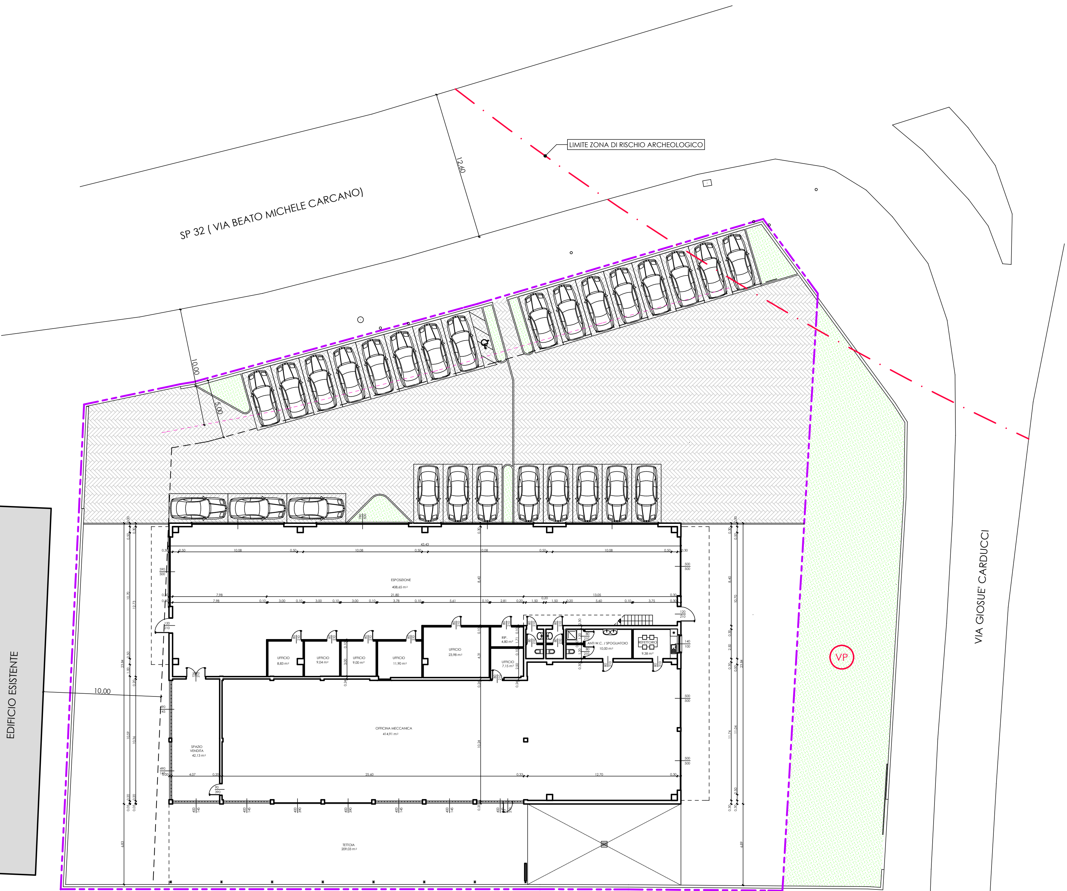
PLANIMETRIA GENERALE PIANO TERRENO
