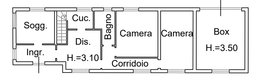
PIANO TERRA - Scala 1:200
