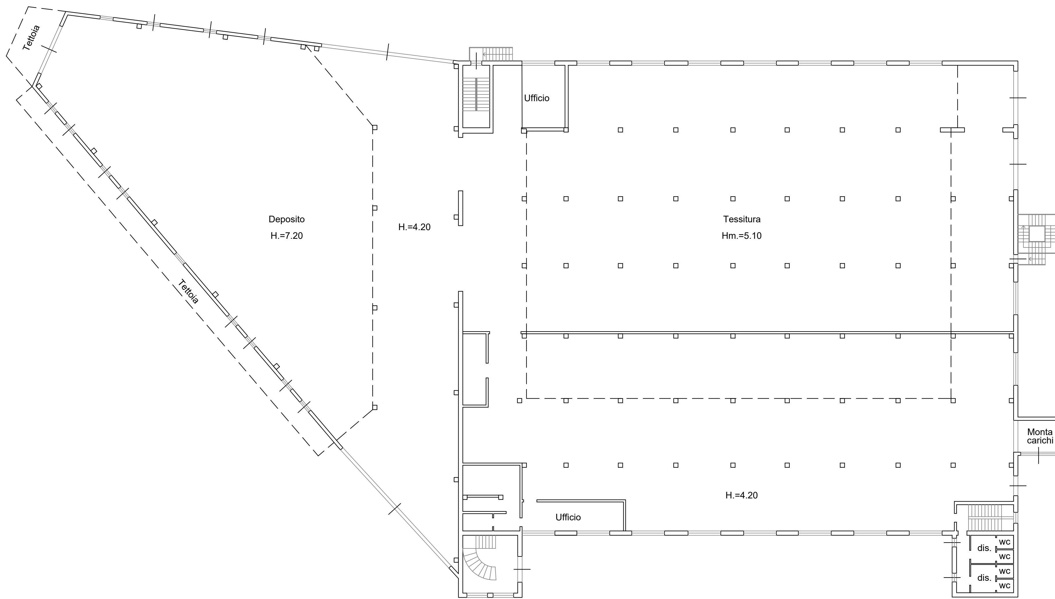
PIANO TERRA - Scala 1:200
