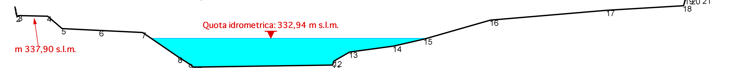
SEZIONE PAI 294 (317) - Progressiva: 63,632 km
