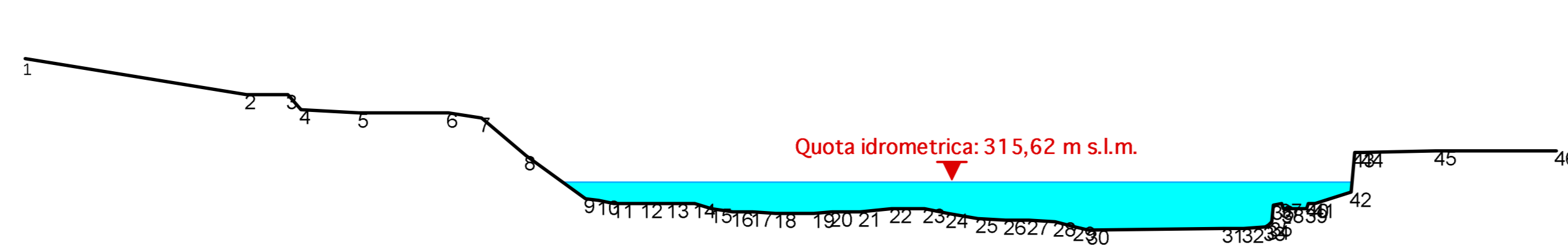
SEZIONE PAI 291 (315) - Progressiva: 64,618 km
