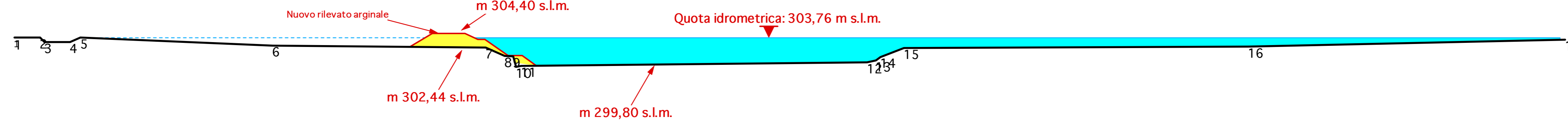
SEZIONE PAI 288 (313) - Progressiva: 65,521 km
