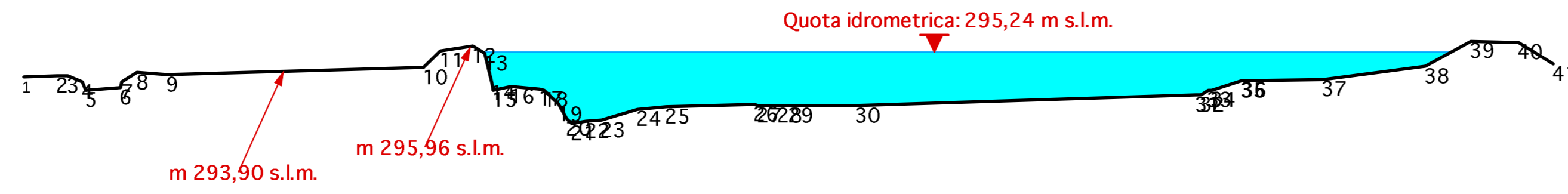
SEZIONE PAI 282 (308) - Progressiva: 68,138 km
