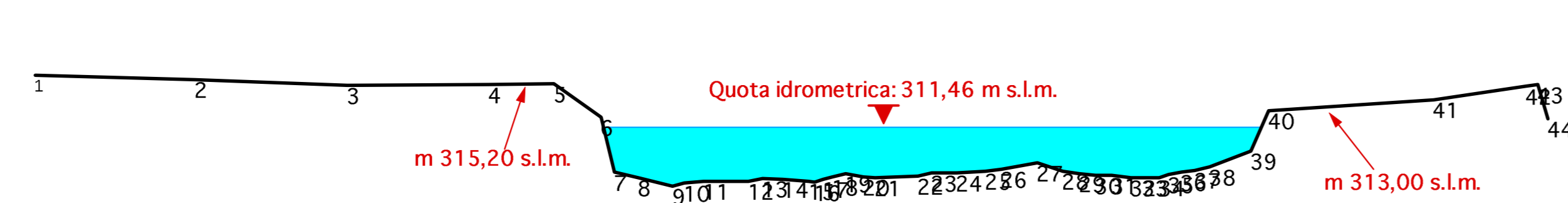
SEZIONE PAI 290 (314) - Progressiva: 65,039 km
