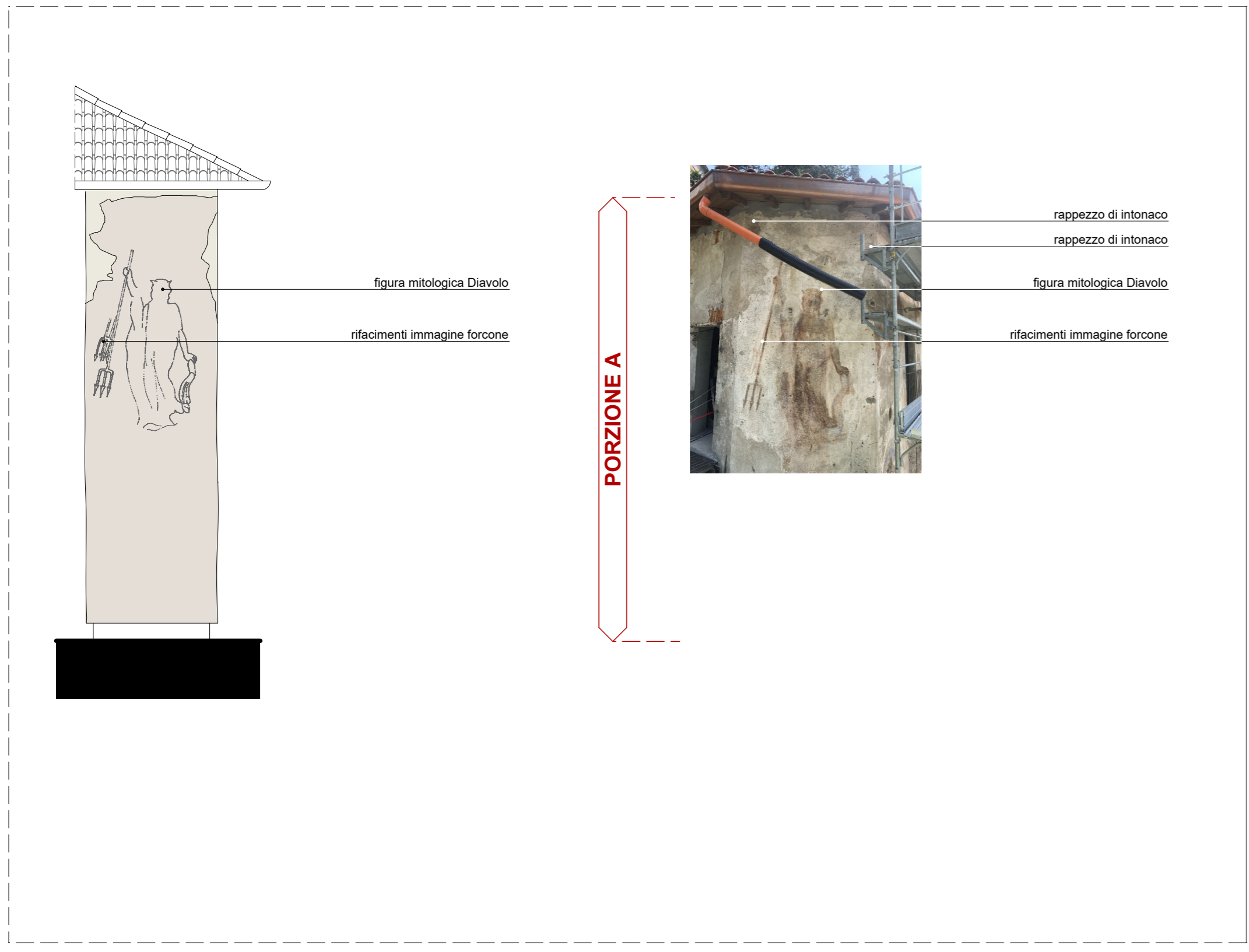
PROSPETTO E-E
